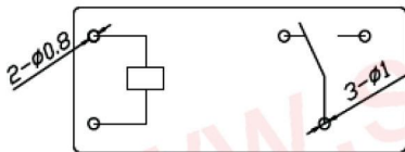
电气原理图
